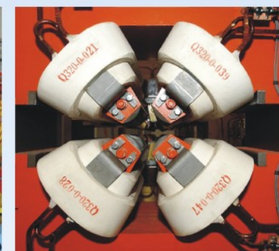
储存环四极磁铁
