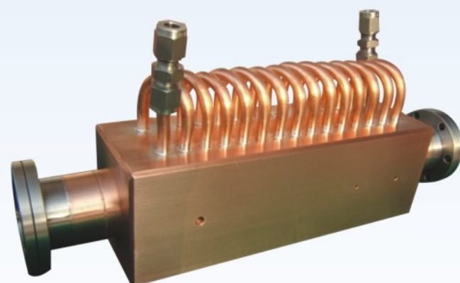
前端区固定光阑
